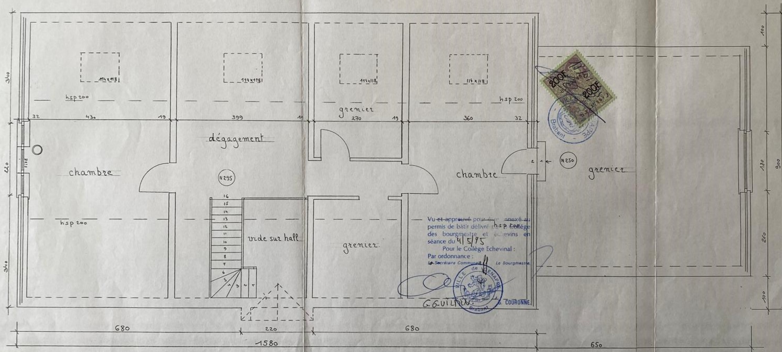
Plan étage 2/100
